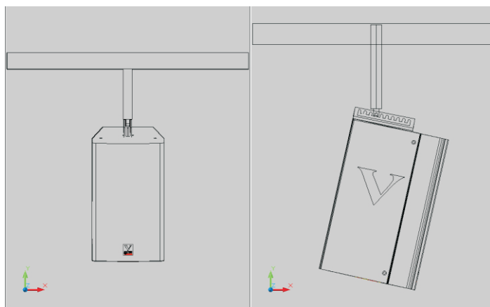
U 型槽专用 吊装方式
